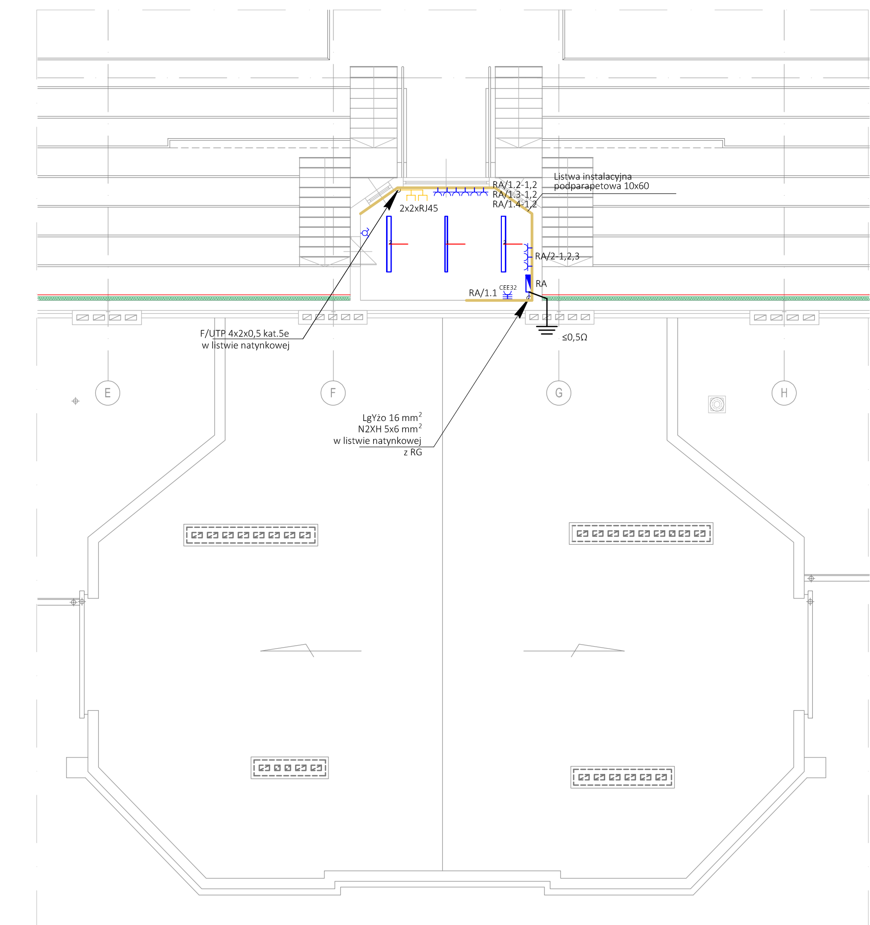
POZIOM TRYBUN
